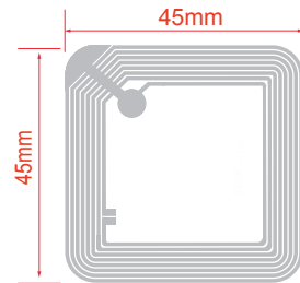
天线图 (Antenna)
